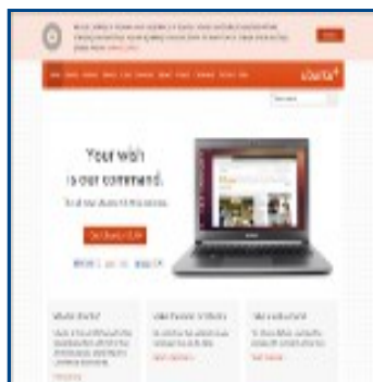
Ubuntu Linux
